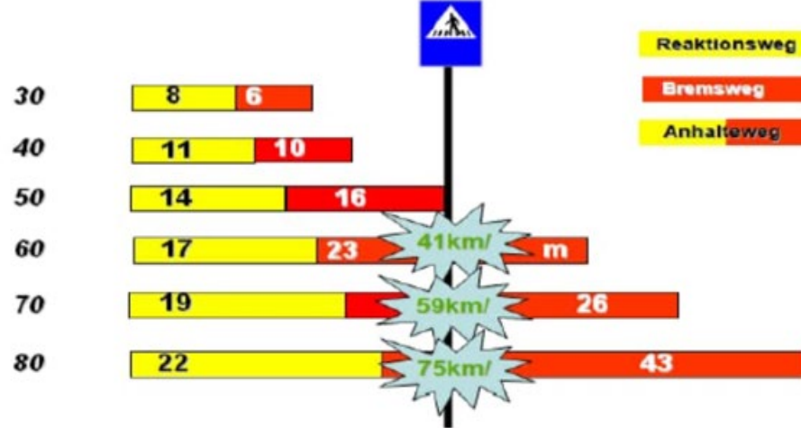
Anhalteweg in Abhängigkeit von der Geschwindigkeit
